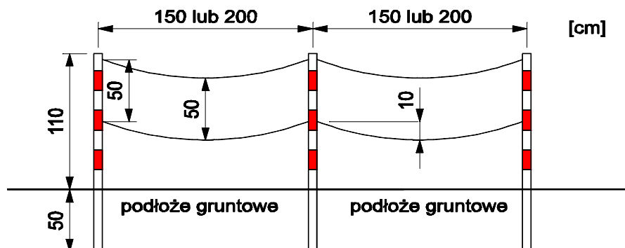
Rys. 1 – przykład ogrodzenia łańcuchowego
